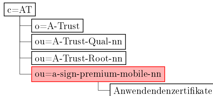
Abbildung 2: A-Trust Verzeichnisbaum
